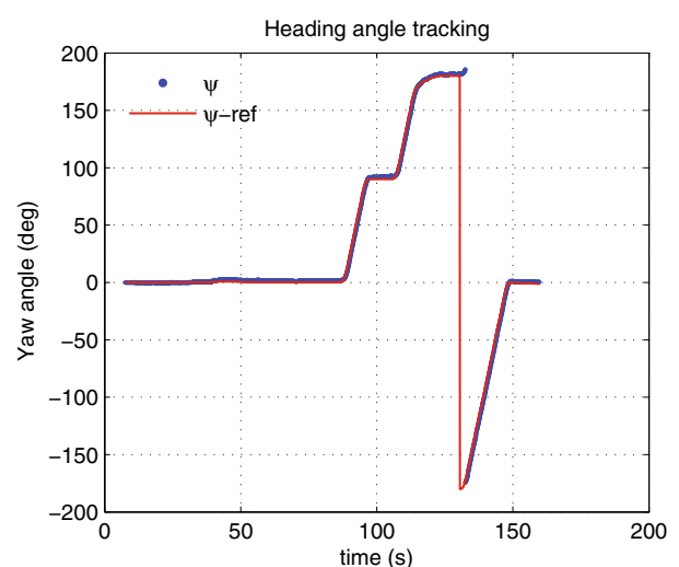
(d) Yaw angle tracking performance
